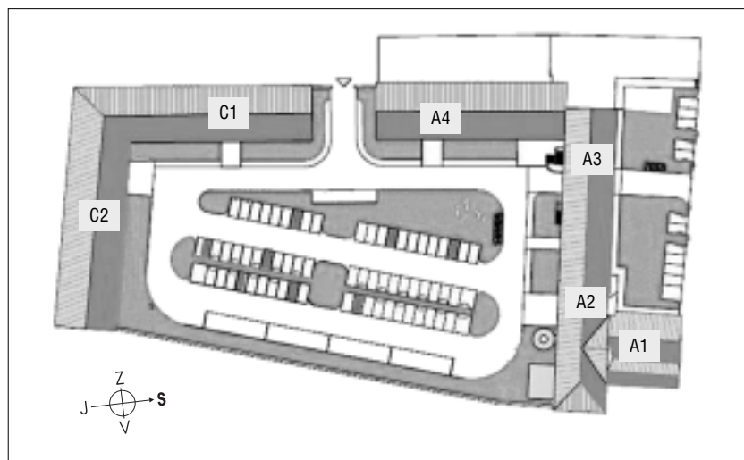
Obr. 4. Schéma areálu hospodářského dvora v Dobrovici (stav po rekonstrukci)
